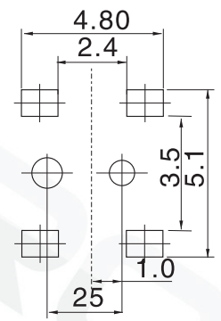
P.C.B 开孔图
